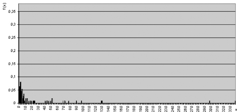
Рис. 1. Функция f_n(x) — нормированная гистограмма распределения числа погибших в терактах
