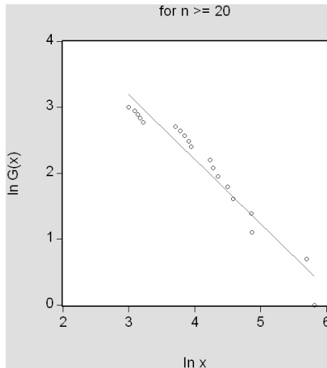
Рис. 2. Кумулятивная гистограмма распределения ущербов от терактов, n = 111
